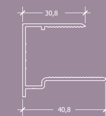
20-25MM 铝型 封口条 U-shaped PC Profile
