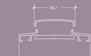
铝型材压条 二件套 AL Cover Profiles
