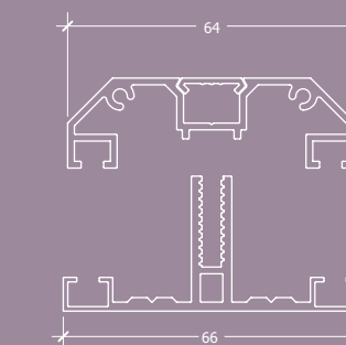
铝型材三件套 AL Triple Profiles
