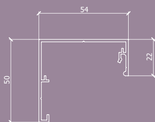
50mm铝型材 上框 LGL40T-AL003 600g/m
