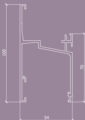
100mm 铝型材连接框 LGL40T-AL004 1420g/m
