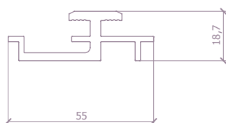
铝型材固定座 LGL40T-AL012
