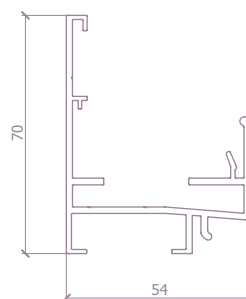
70mm铝型材 底框 LGL40T-AL008 1085g/m
