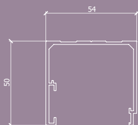
50mm铝型材 单体上框 LGL40T-AL010 850g/m
