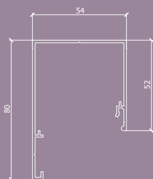
80mm铝型材 上框 LGL40T-AL002 850g/m
